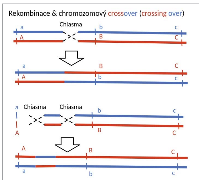
Obrázek 6. Chromozomové rekombinace
